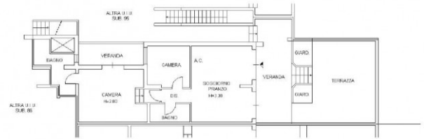
PIANTA PIANO TERRA Hm=3.00
