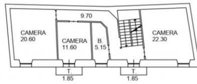
PIANO PRIMO H= m. 3.50
